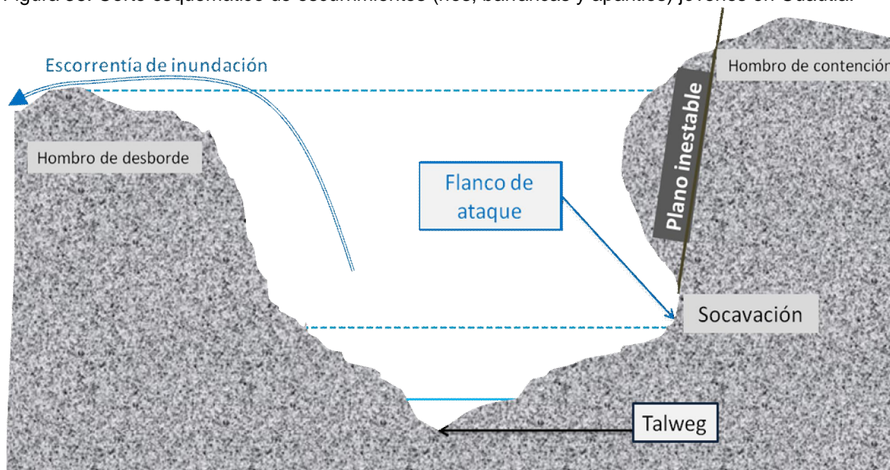
Figura 35. Corte esquemático de escurrimientos (ríos, barrancas y apantles) jóvenes en Cautla.
