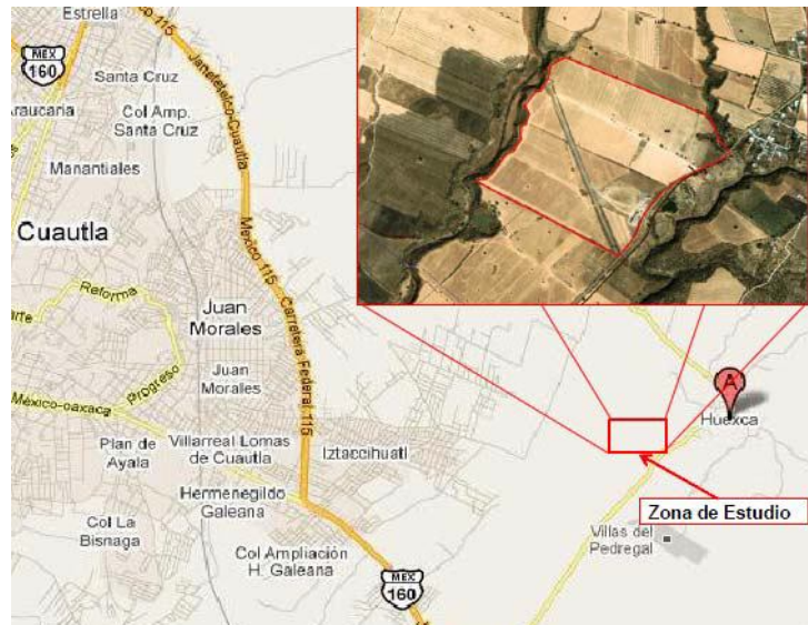
FIGURA 13. UBICACIÓN DE LA NUEVA CENTRAL DE CICLO COMBINADO "264 CC CENTRO MORELOS", (FUENTE TRANSCONSULT S.C.)
